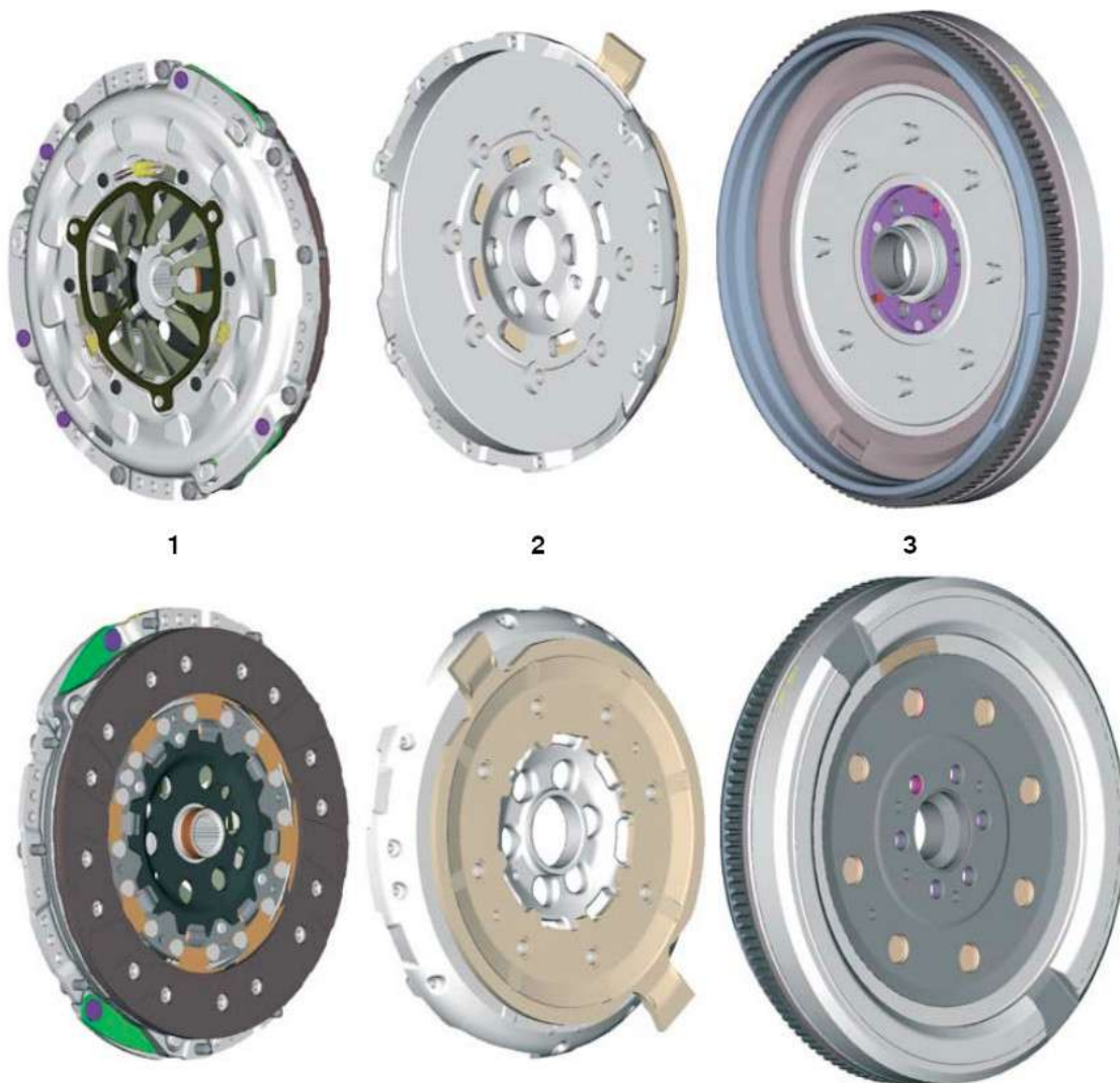
Демпферная муфта маховика (DMF) – вид спереди и сзади
