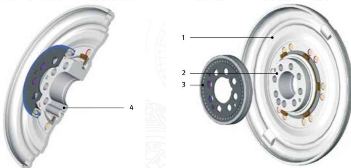
Стандартный двухмассовый маховик (DMF) – размер подшипника
