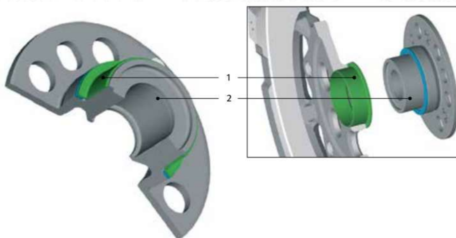
Стандартный двухмассовый маховик (DMF) – плоский подшипник скольжения
