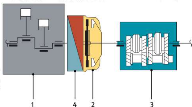
Принцип работы традиционного маховика
