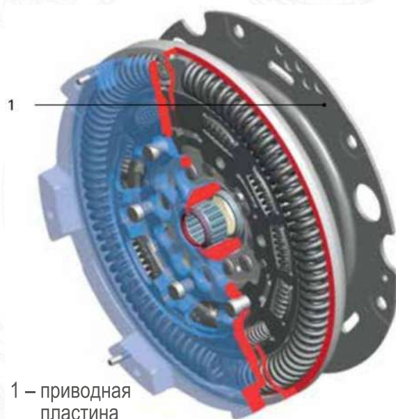
DMF с приводной пластиной
