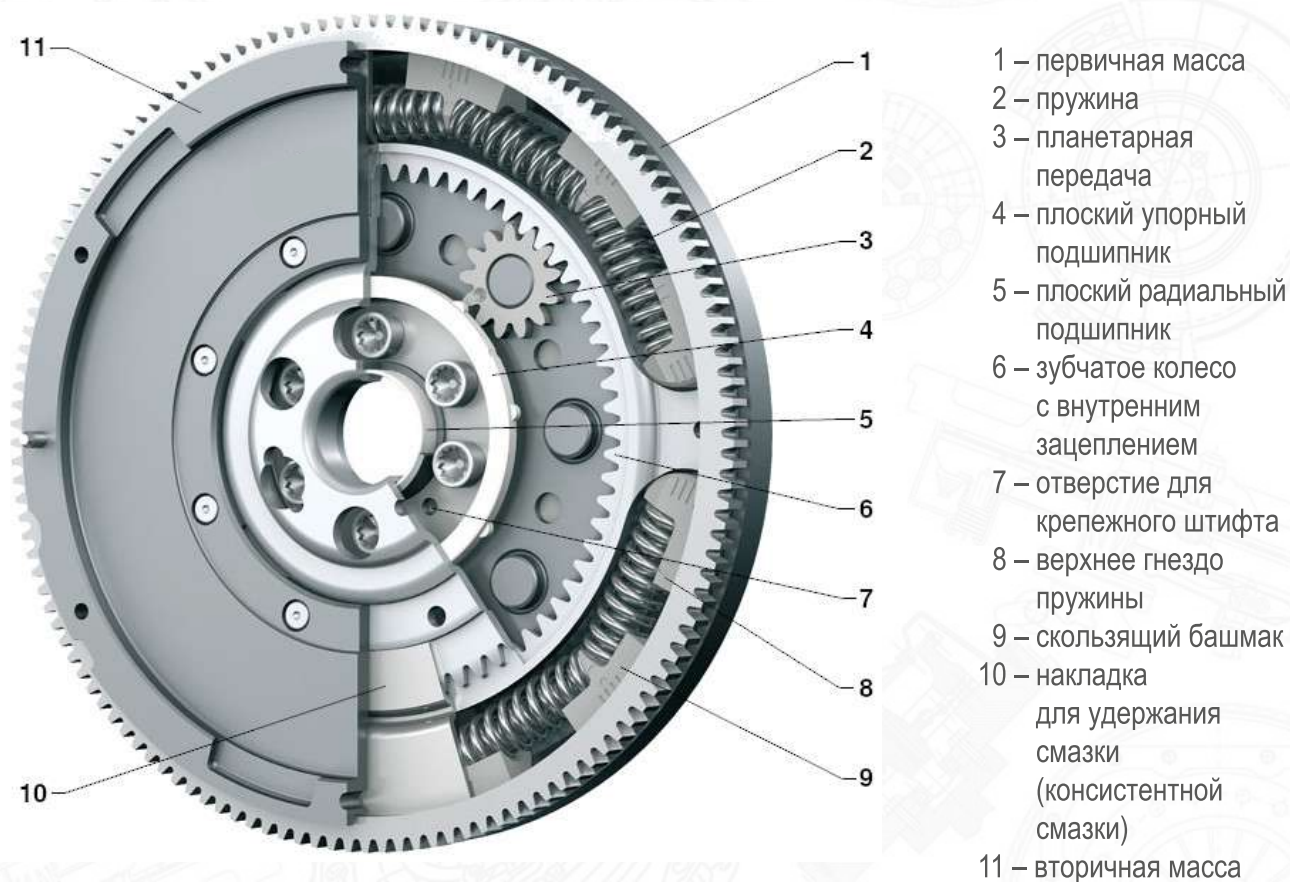
DMF с планетарной передачей
